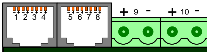
Рисунок 3 – Сторона портов общего назначения
