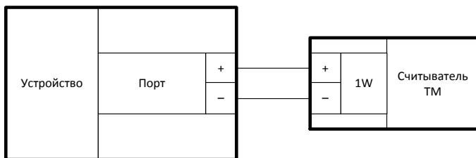
Рисунок 14 – Схема подключения считывателя ключей
