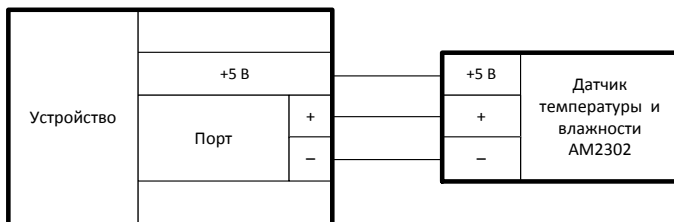
Рисунок 17 – Схема подключения датчика температуры и влажности
