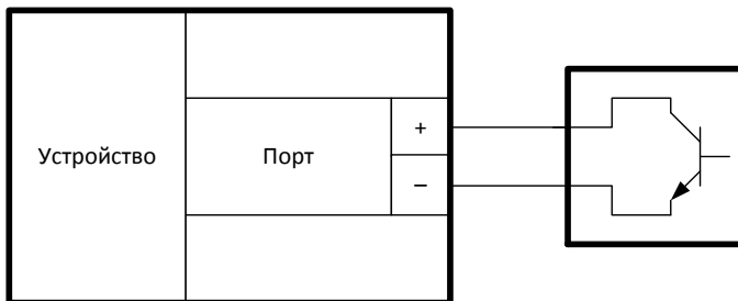
Рисунок 8 – Подключение датчика с выходом типа «Открытый коллектор»
