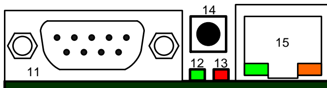
Рисунок 4 – Сторона интерфейсов и питания
