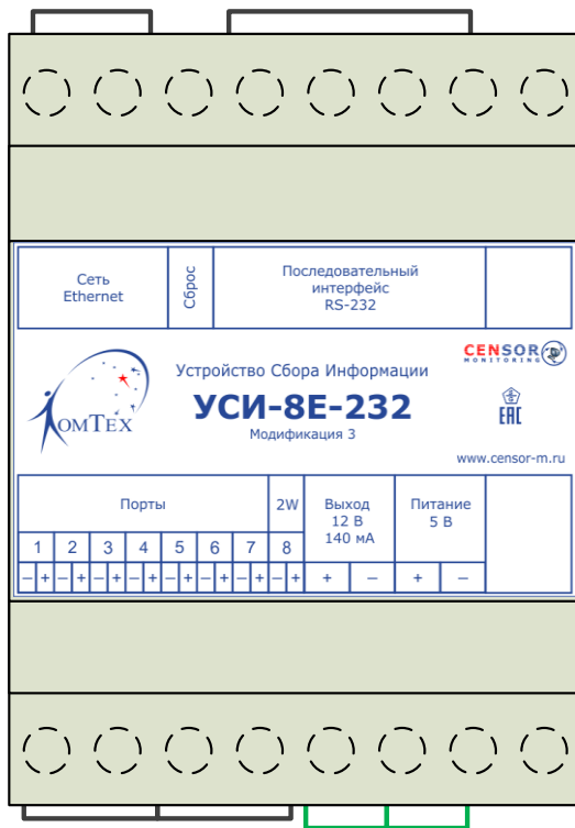
Рисунок 1 – Внешний вид Устройства
