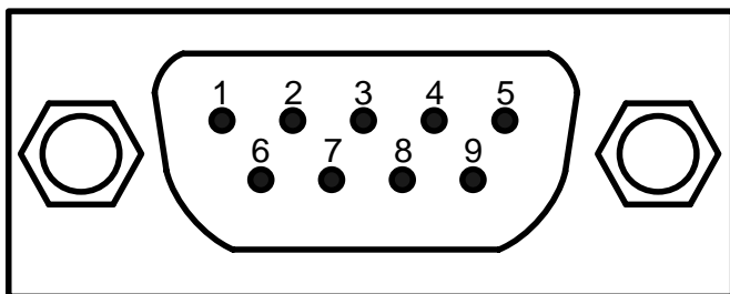
Рисунок 19 – Разъем последовательного интерфейса
