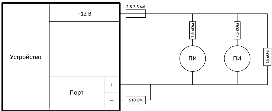
Рисунок 18 – Схема подключения пожарного шлейфа
