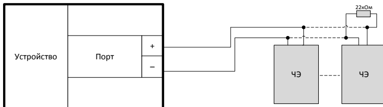
Рисунок 15 – Подключение шлейфа затопления
