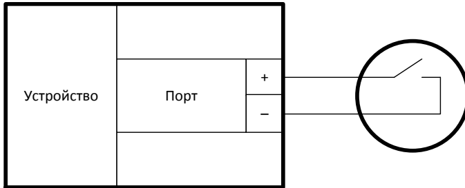
Рисунок 6 – Подключение датчика с выходом типа «Сухой контакт»
