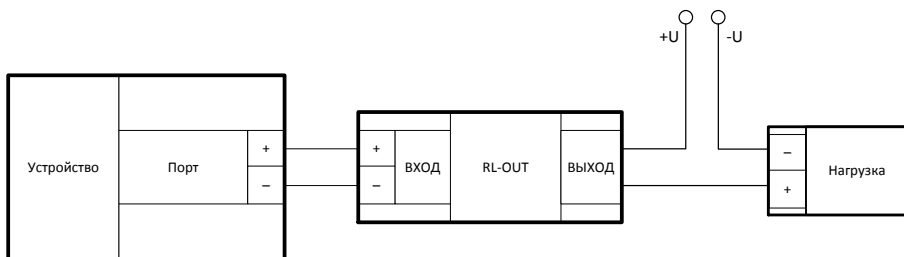
Рисунок 12 – Подключение модуля RL-OUT
