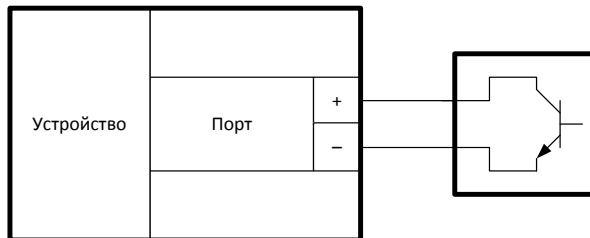
Рисунок 6 - Подключение датчика с выходом типа «Открытый коллектор»
