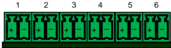
Рисунок 3 – Нижняя сторона Устройства
