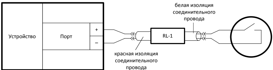
Рисунок 8 - Подключение датчика с помощью модуля RL-1
