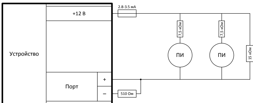
Рисунок 18 - Схема подключения пожарного шлейфа
