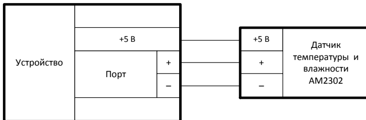
Рисунок 17 - Схема подключения датчика температуры и влажности
