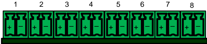
Рисунок 5 – Нижняя сторона Устройства
