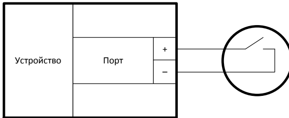
Рисунок 7 - Подключение датчика с выходом типа «Сухой контакт»
