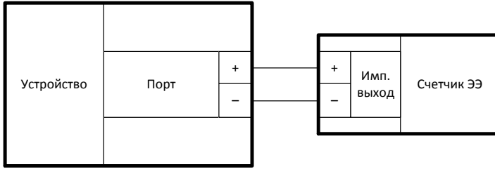
Рисунок 11 - Подключение импульсного выхода счетчика электроэнергии
