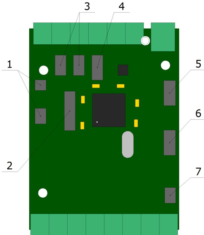
Рисунок 2 - Расположение разъемов для подключения функциональных модулей
