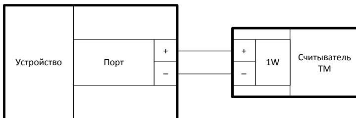
Рисунок 14 - Схема подключения считывателя ключей
