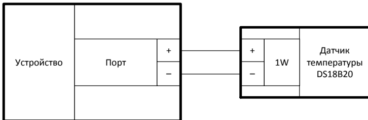
Рисунок 13 - Схема подключения датчика температуры
