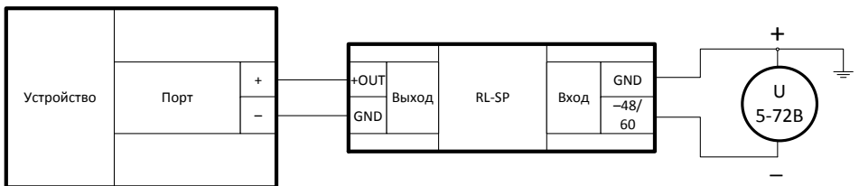
Рисунок 10 - Подключение модуля RL-SP для измерения напряжения
