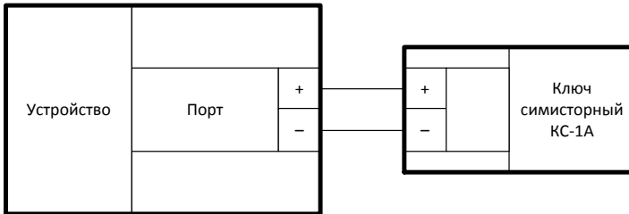
Рисунок 12 - Подключение управляемой розетки
