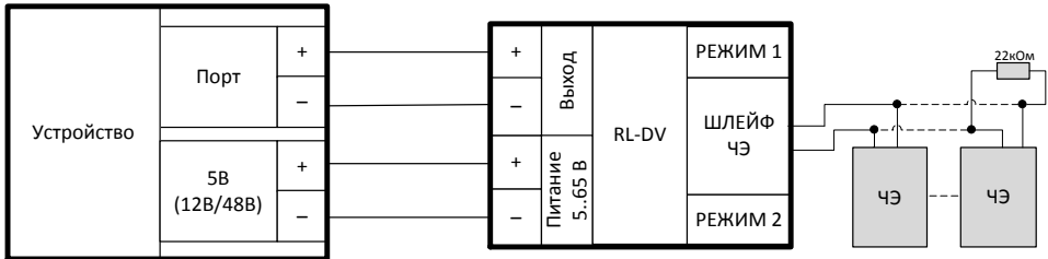
Рисунок 16 - Подключение шлейфа затопления через RL-DV
