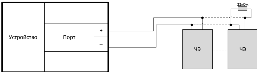
Рисунок 15 - Подключение шлейфа затопления
