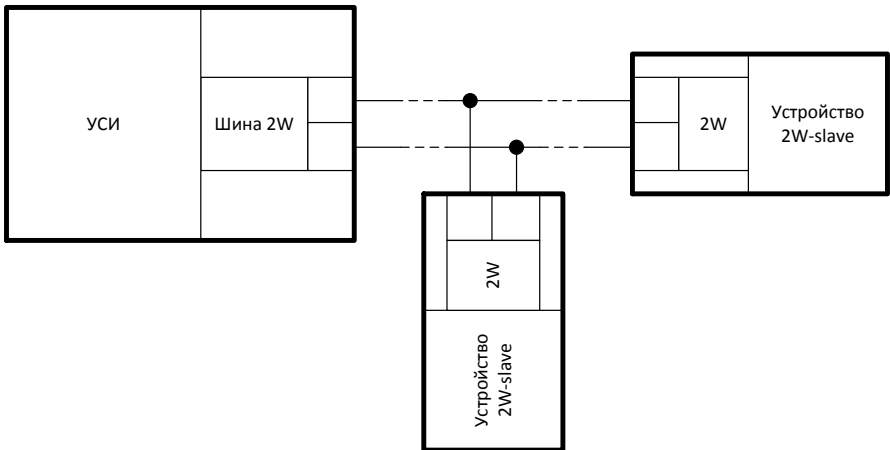
Рисунок 6 – Подключение 2W-slave устройств
