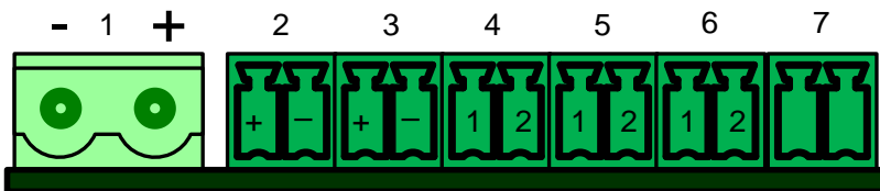
Рисунок 3 – Верхняя сторона Устройства
