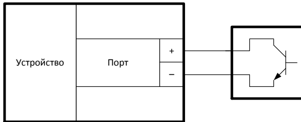
Рисунок 9 - Подключение датчика с выходом типа «Открытый коллектор»
