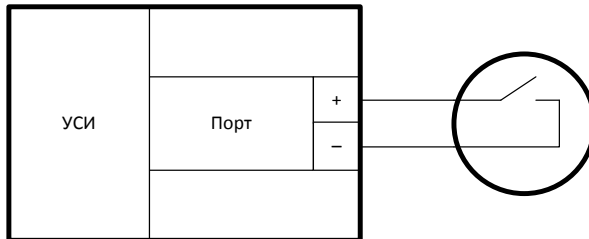
Рис. 4. Подключение датчика с выходом типа «Сухой контакт»
