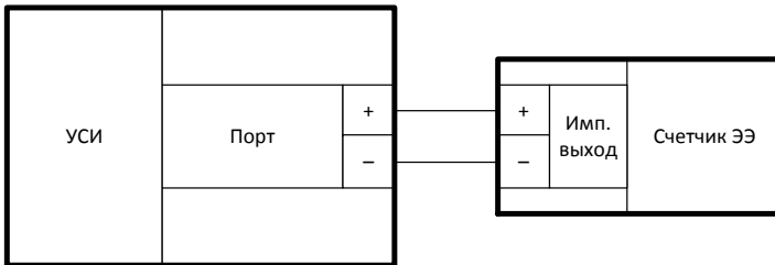
Рис. 6. Подключение импульсного выхода счетчика электроэнергии.
