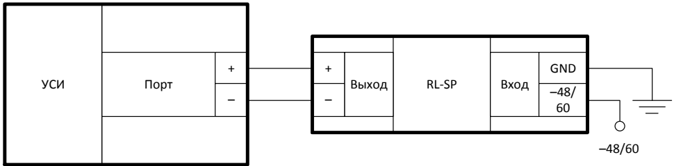
Рис. 9. Измерение стационарного напряжения.
