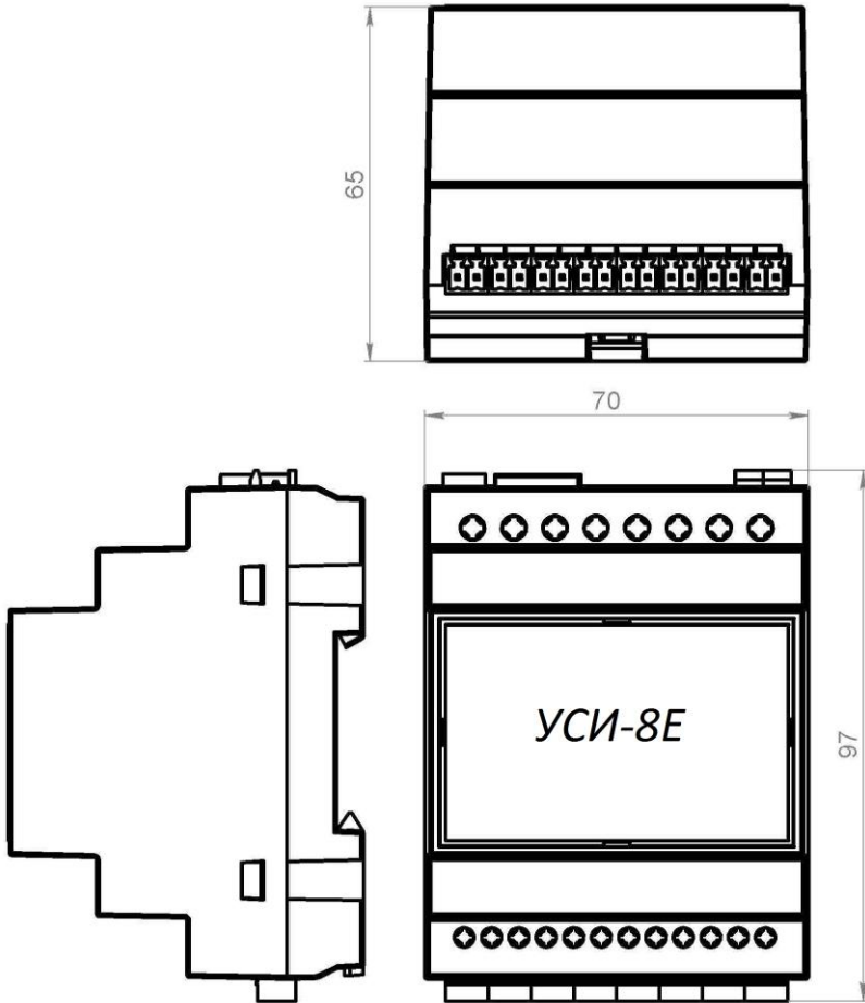
Рис. 1. Габаритные размеры
