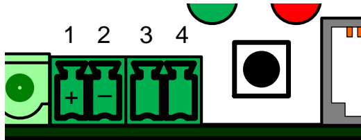
Рис. 12. Разъем последовательного интерфейса
