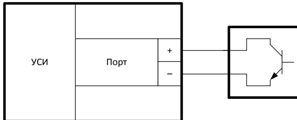
Рис. 5. Подключение датчика с выходом типа «Открытый коллектор»
