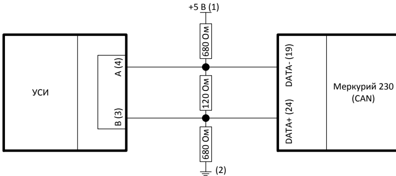
Рис. 13. Подключение счетчика электроэнергии Меркурий 230 (CAN) Цифрами в скобках обозначены номера контактов разъемов на устройствах, соответствующие данным сигналам.
