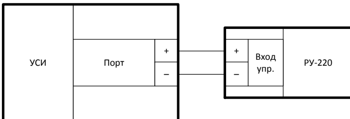
Рис. 7. Подключение управляемой розетки.
