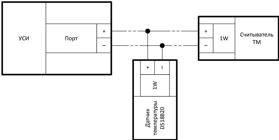
Рис. 8.Схема подключения устройств 1W.
