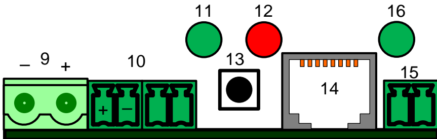
Рис. 3 Верхняя сторона устройства
