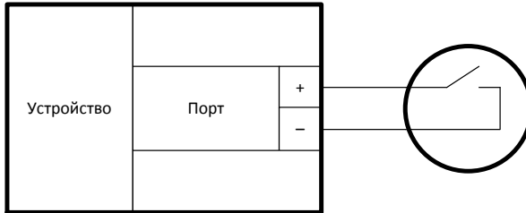
Рисунок 7 - Подключение датчика с выходом типа «Сухой контакт»
