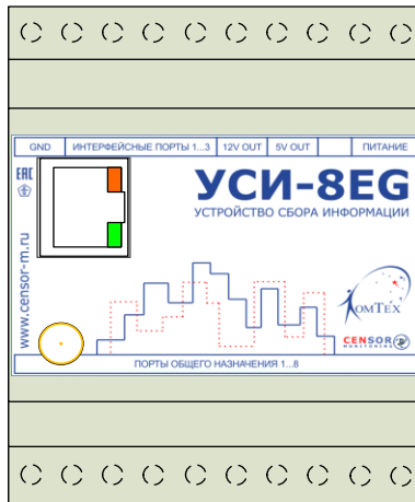
Рисунок 1 – Внешний вид Устройства сбора информации USI-8EG
